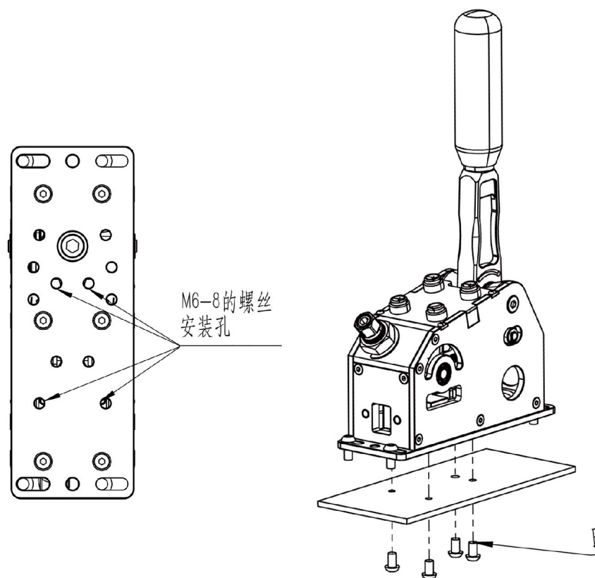
B. 圆头螺丝M6-8 X 4
